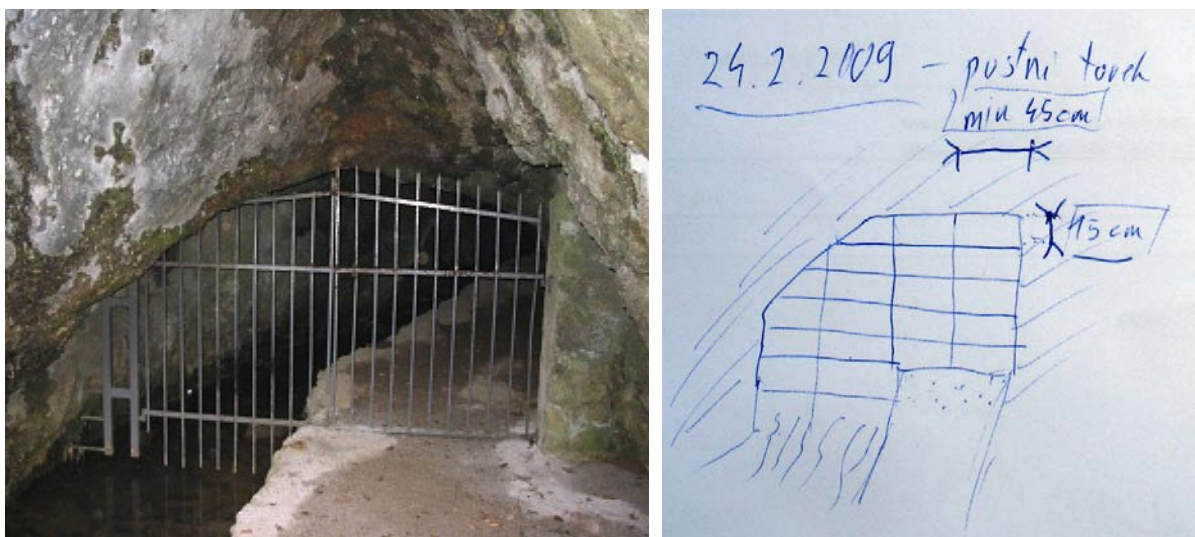
Slika 8. a) Sedanje rešetke na vhodu Pekla pri Zalogu (foto. P. Presetnik, 23.2.2005) in b) terenska skica predloga nove oblike rešetk.
