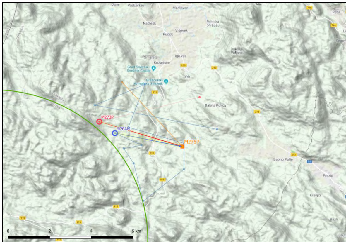
Slika 18: Vzorci križancev med volkom in psom, zaznanih v vzorčenjih 2016/17 in 2017/18. Puščica kaže starševstvo, črte povezujejo v kronološkem zaporedju vzorce istega osebk. Gre za starša in potomca (potomec se je pojavil v sezoni 2017/18). Pri enem staršu in enem potomcu je izbira kateri je starš in kateri potomec arbitrarna. Glede na čas pojavljanja in delež volčjega/pasjega predništva je verjetno M20AM oče.
