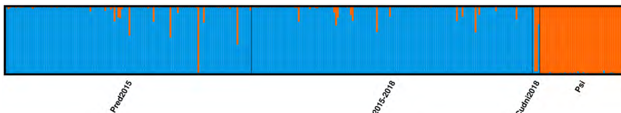
Slika 17: STRUCTURE graf križanja med volkom in psom. Več živali kaže znake pasjega predništva, vendar lahko samo pri treh osebkih iz trenutnega vzorčenja z gotovostjo govorimo o križancih. V grafu sta vidna še dva križanca, zaznana v 2012 in en zaznan v 2014.
