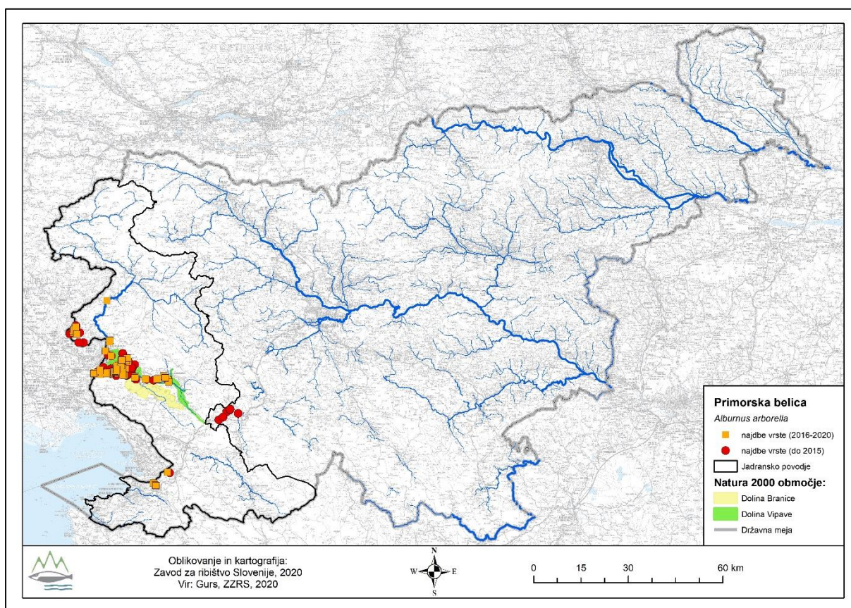
Slika 3: Razširjenost primorske belice v Sloveniji. Oranžni kvadrati prikazujejo najdbe vrste v poročevalskem obdobju 2016 – 2020, rdeče pike pa najdbe vrste pred tem obdobjem.
