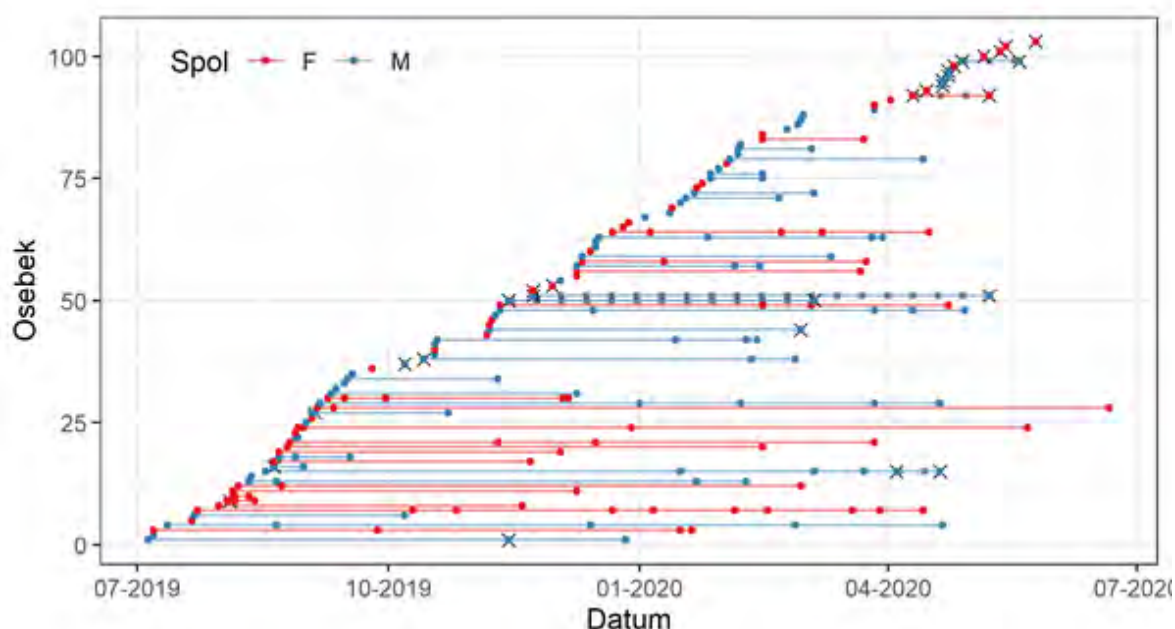
Slika 21: Saturacijski graf označevanja / ponovnega ulova za genetski monitoring volkov v Sloveniji v sezoni 2019/2020. Vsaka vodoravna črta je osebek, vsaka pika vzorec. Osebkovi vzorci so kronološko razporejeni glede na prvi »ulov« (najdba prvega vzorca).
